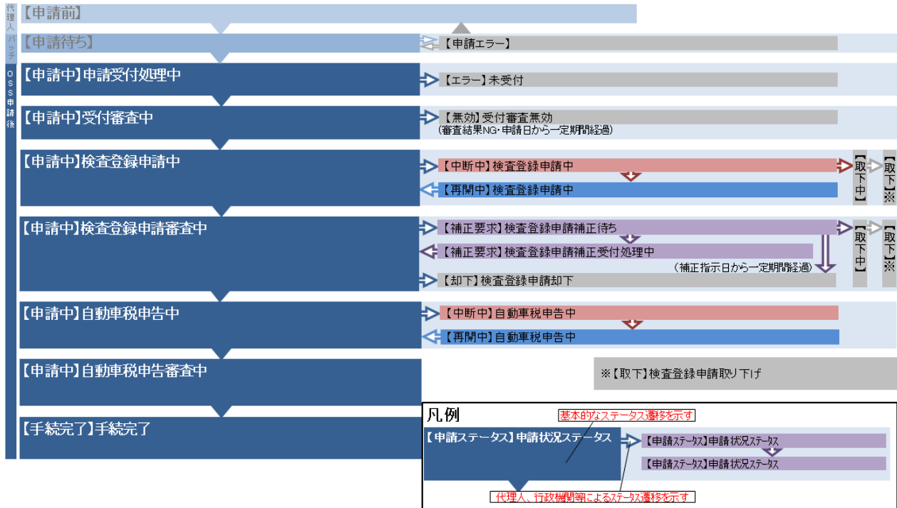
図 1-1 OSS 申請の流れ(ステータス遷移及び利用機能一覧)
