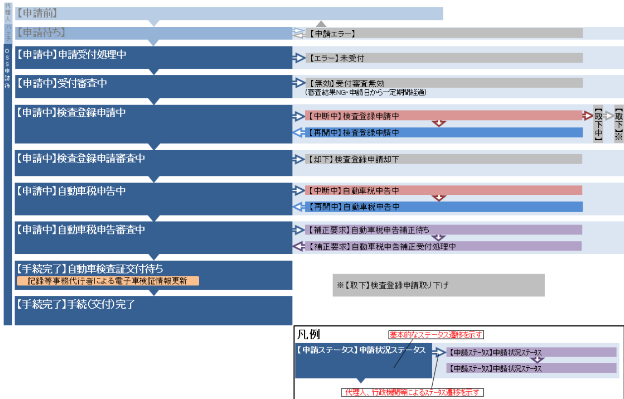
図 1-1 OSS 申請の流れ(ステータス遷移及び利用機能一覧)
